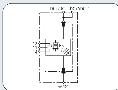
Schema di principio DSE M 1 ... (FM)
