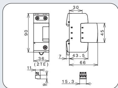
Dimensioni DSE M 1 ... (FM)
